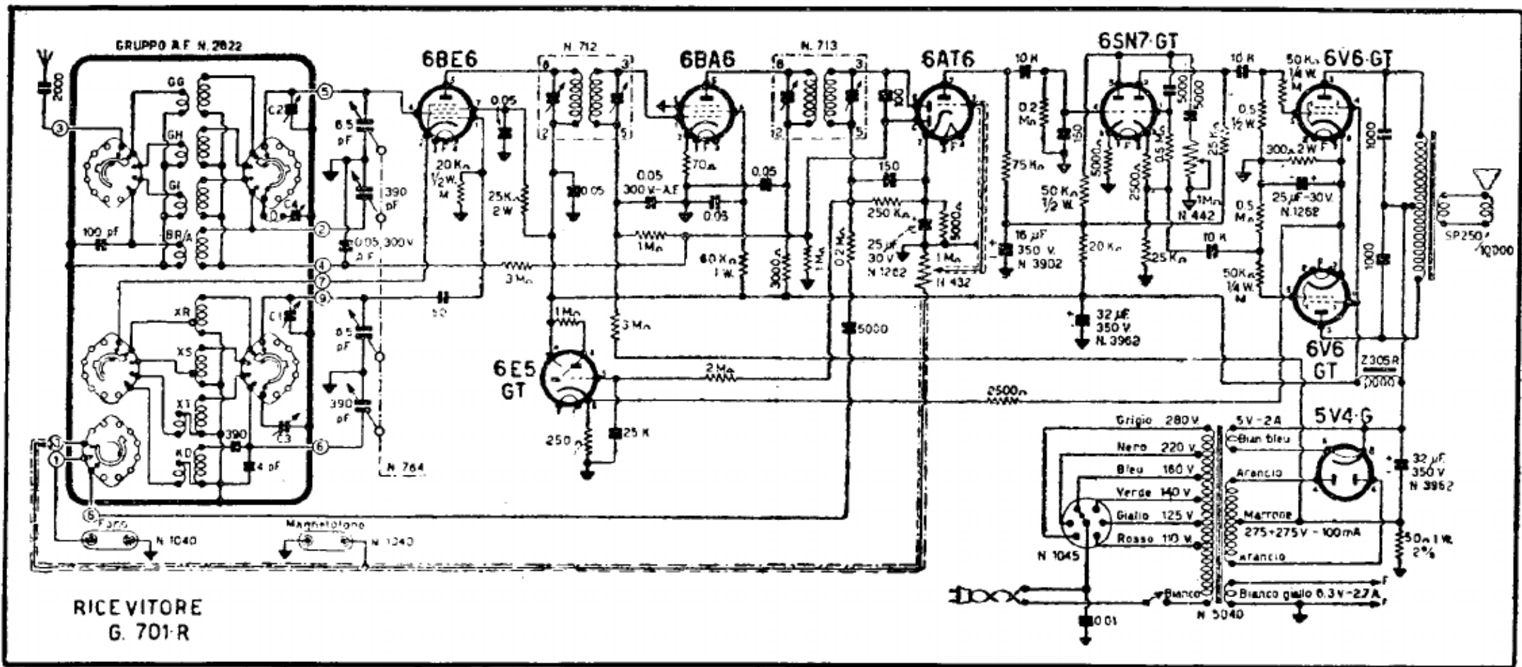
GELOSO - Mod. Super G 701. Onde medie da 190 a 580 m. e sei bande allargate di 16, 19, 25, 31 e 50 m. Media frequenza 467 kc/s. Sensibilità MF 20 microvolt. Potenza d'uscita 8 watt.
